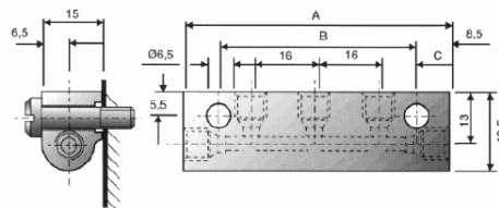
编号 42426 5孔双边分油块
