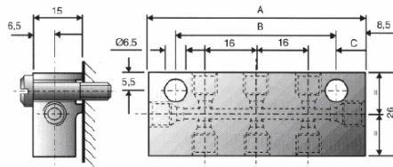
零件编号 4 编号 42426 8孔双边分油块
