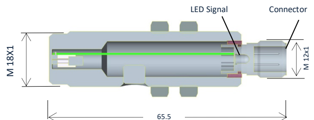
1655326 ULTRASENSOR M18x1
