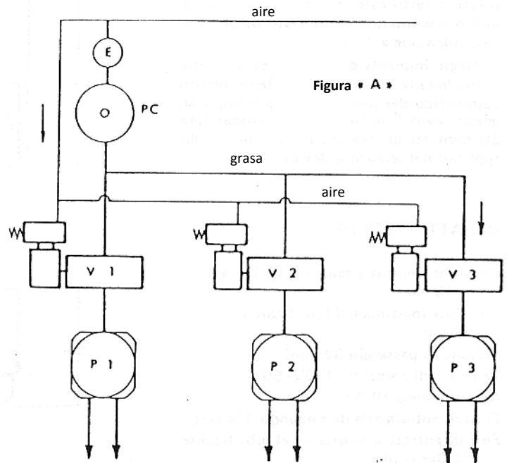
Esquema eléctrico de válvulas electro neumáticas en un tipo de aplicación (fig. A)
