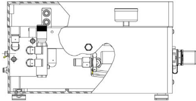
SEZIONE C-C
